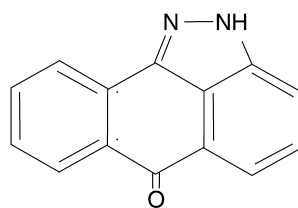
SP600125
